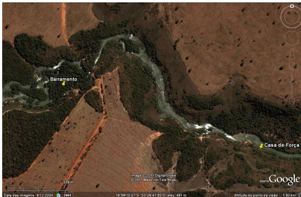
Figura 2 – Vista da PCH e do vale, em 2010
