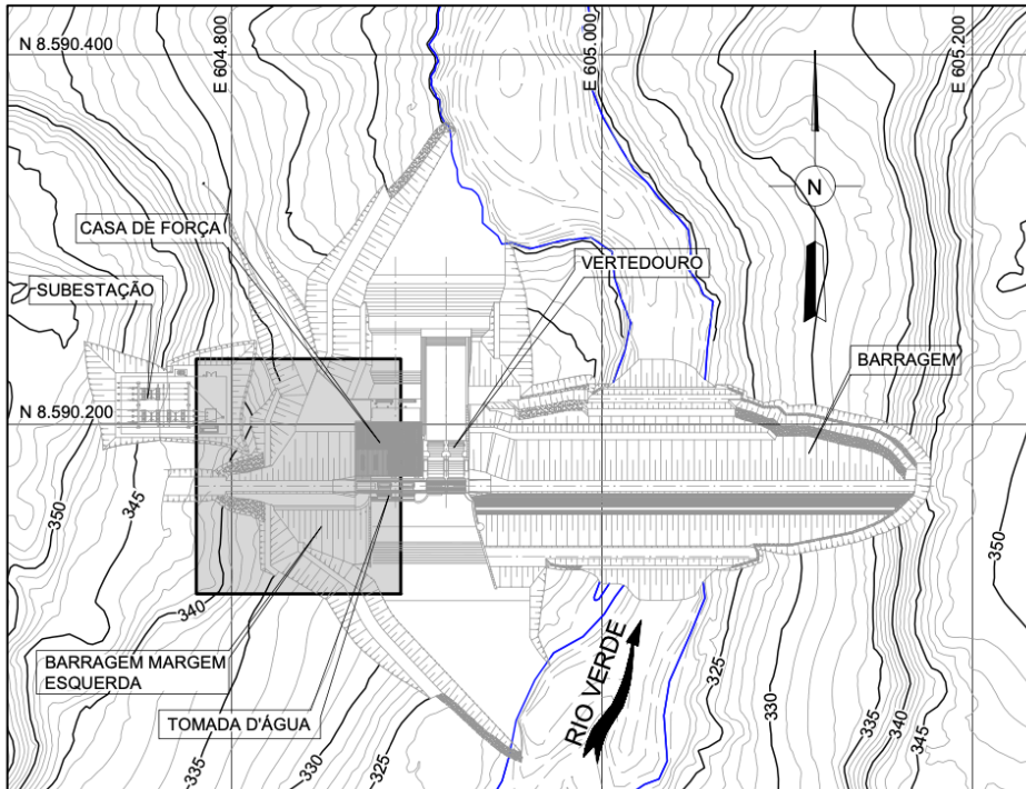
Figura 4 – Arranjo geral da PCH Foz do Cedro
