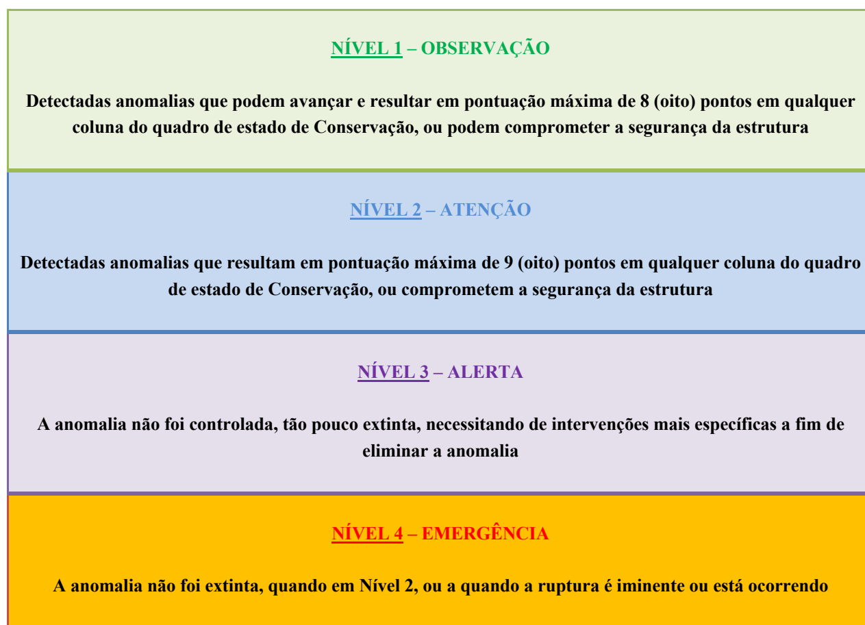
Figura 11 – Níveis de Alerta da Barragem da PCH Foz do Cedro
