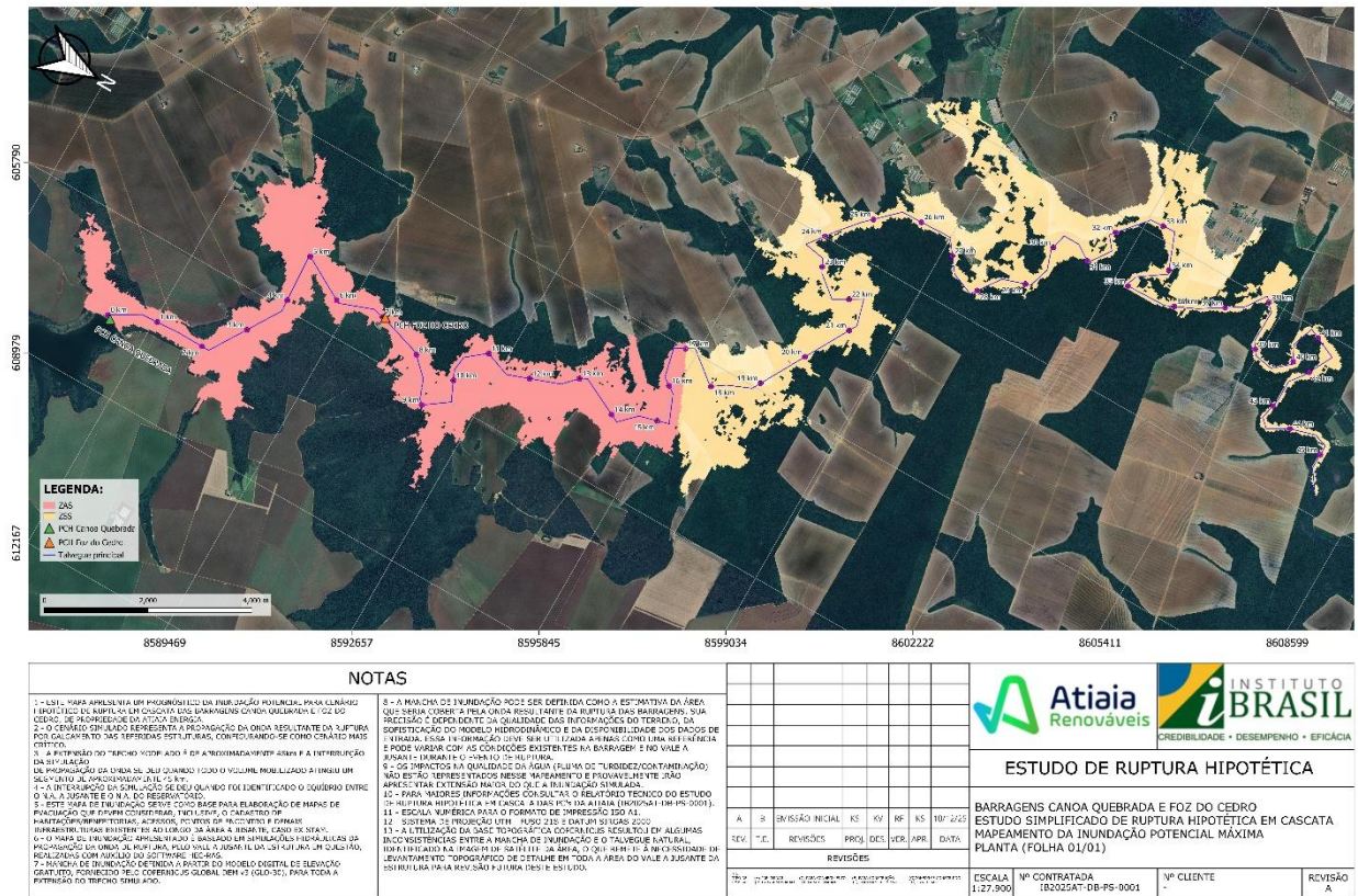
Figura 3 - Zonas de Autossalvamento e Zonas secundárias
